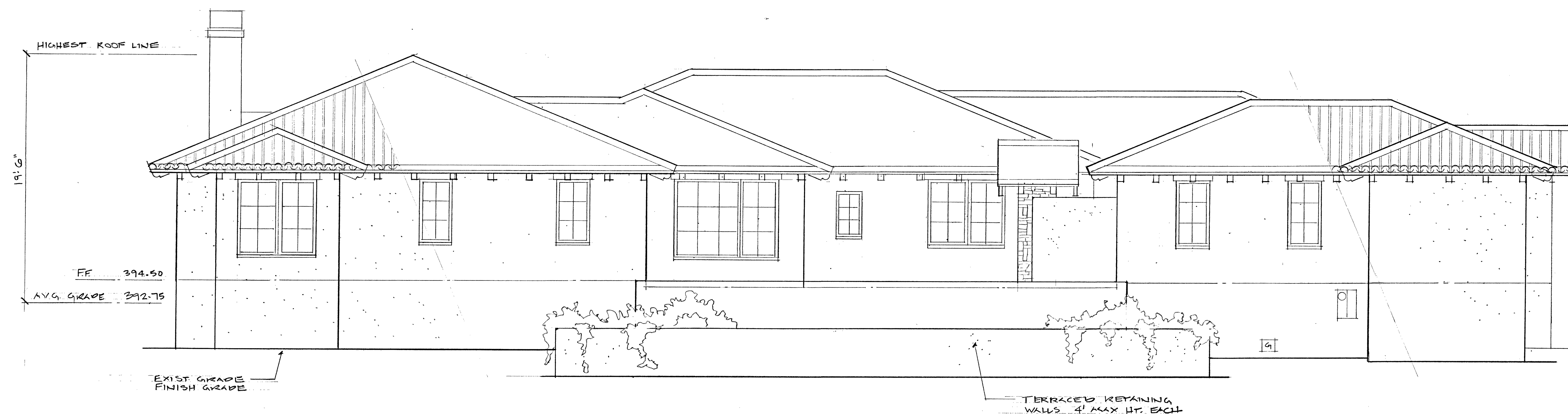
S O U T H E L E V A T I O N
