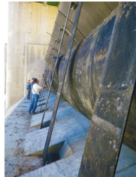
Inflated Nacimiento Spillway rubber dam
