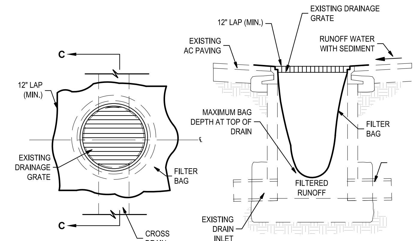
5 DI PROTECTION TYPE 3 - GRAVEL BAG DETAIL (SE-10) SCALE: NTS
